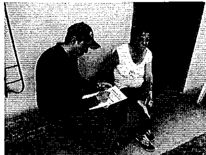
Fotografía 1. Visita, recorrido, aforamiento en el Canal de Riego Predio Batallas.
