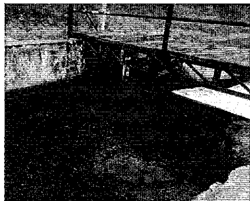
Fotografía 7. Entrada de agua cruda al Presedimentador de la Planta EAPA San Mateo.
