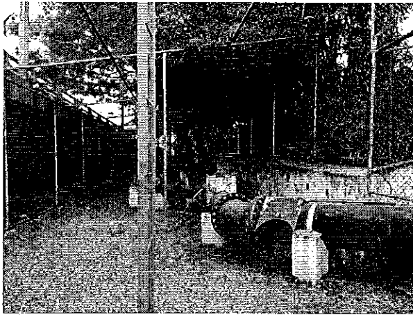
Fotografía 3. Macromedidor Sur, sector de ingreso del agua importada de AMAGUA, Samborondón
