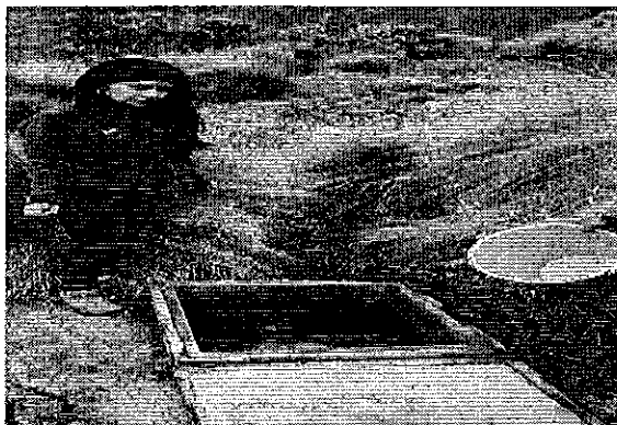
Ilustración 1. Determinación del Caudal, aforo volumétrico, en tanque rompe presiones JAAP Juan Montalvo del Cantón Cayambe.
