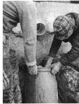
Fotografía 6. Aforo de la captación de agua del brazo derecho de la Quebrada Dos Chorreras (en dirección del flujo del agua) para piscícola del Sr. Pedro León.
