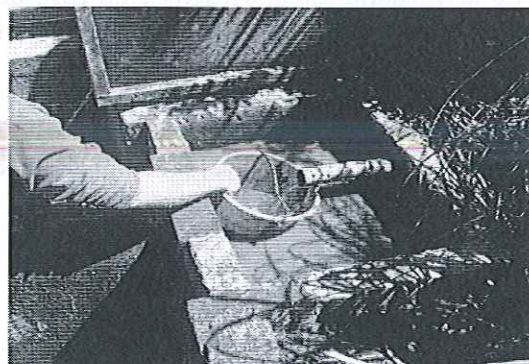
Fotografía 2. Medición de caudal por método volumétrico en caso Cochasqui.
