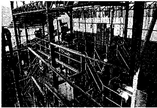
Fotografía 1.-Planta de procesamiento del mineral
