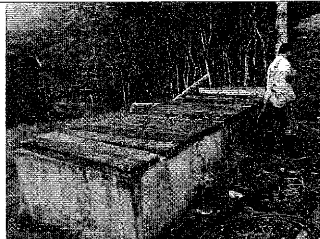
Ilustración 8. Desarenador -- sistema de agua Potable de Santa María del Toachi.
