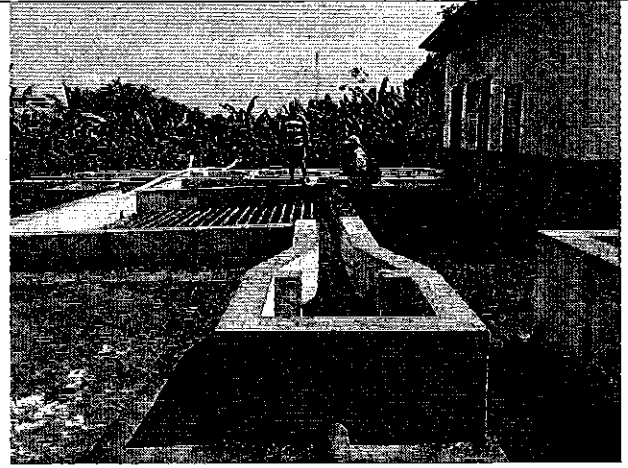
Ilustración 6. Planta de tratamiento para agua potable del sistema de Puerto Limón.
