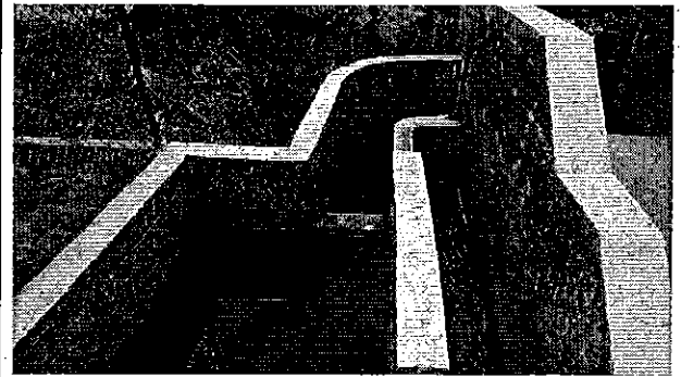
Fotografía 2.- Captación de agua Proyecto Minero Loma Larga.
