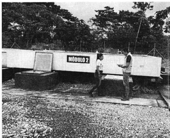
Fotografía 3. Inspección sedimentadores – planta de tratamiento de agua potable GADM- Putumayo
