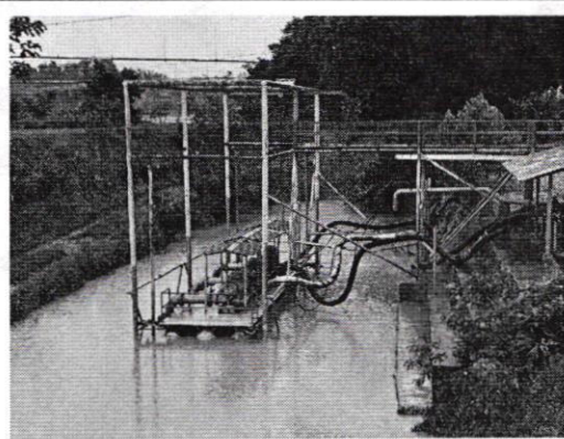
Fotografía 3. Fuente de agua de EMAPALA.
