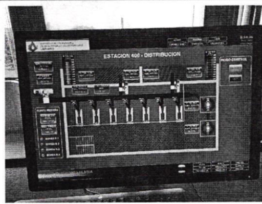
Fotografía 5. Sistema SCADA EMAPALA.
