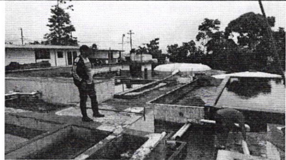
Fotografía 6. PTAP Valle Alto, sistema Cumandá.
