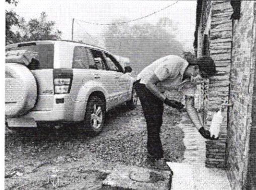
Fotografía 10. Toma de muestra de agua último punto Red Sistema Cumandá.
